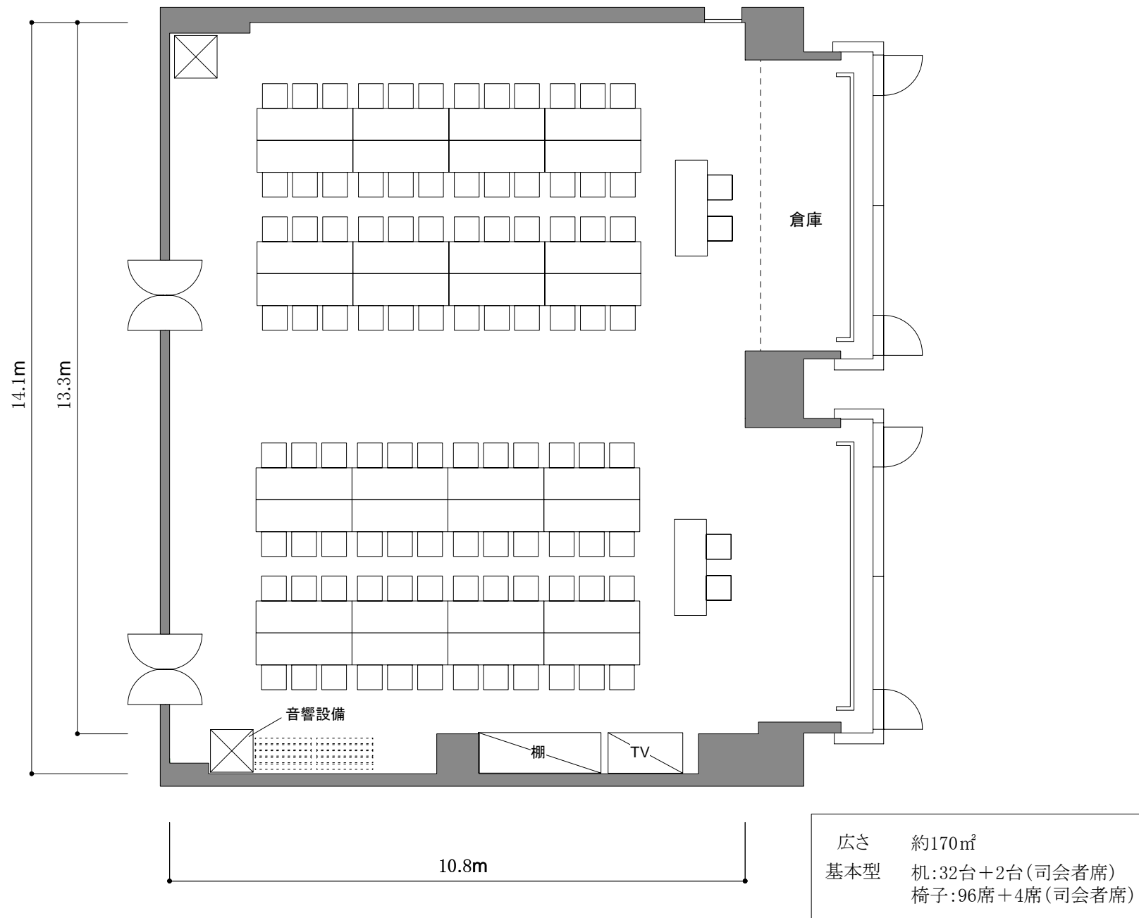
第5・6集会室（高砂・羽衣一間仕切りなし）平面図（S=1：100）
